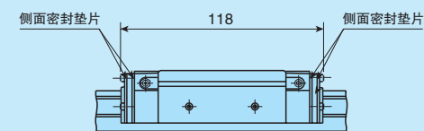
图2 附带双层密封垫片的滑块的尺寸(大小尺寸25) (辅助标记 /V /VV)
