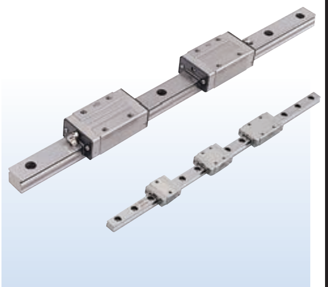
照片所示为特殊环境用密封垫片(/RE)和钢制侧板(/BS)的搭配。
