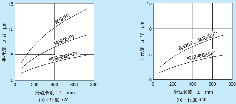
图1.1 LWLM的滑轨的平行度
